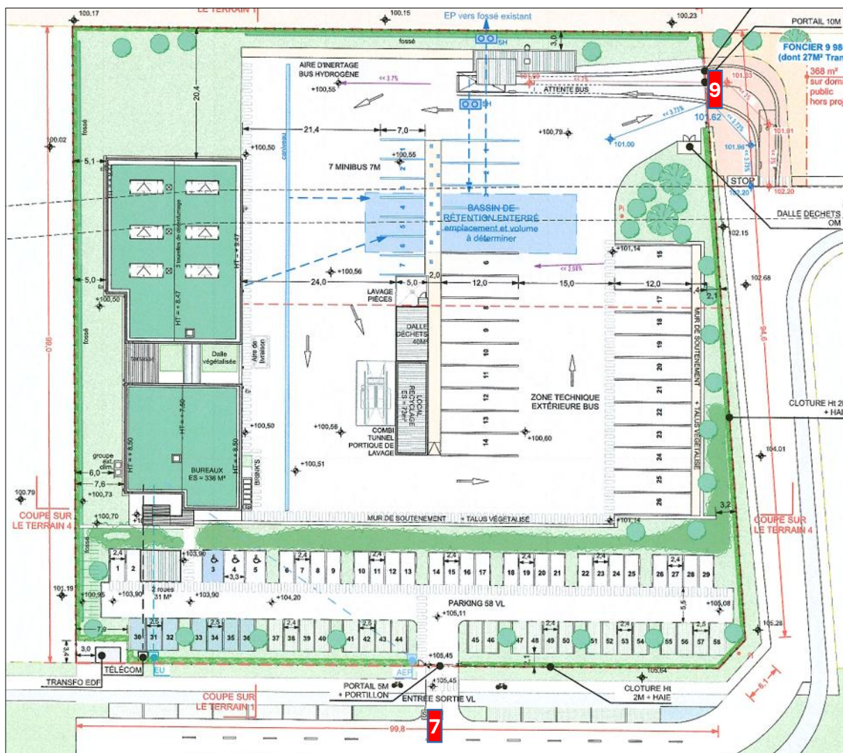
Plan de masse du projet de construction – PC 89 024 24 00019
